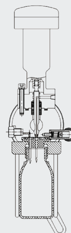
针插式
