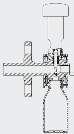
侧装式
