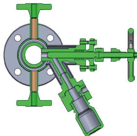
根据客户的需求定制Y型保温截止式取样阀
