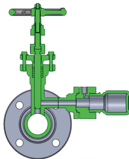
基本型截取式取样阀
